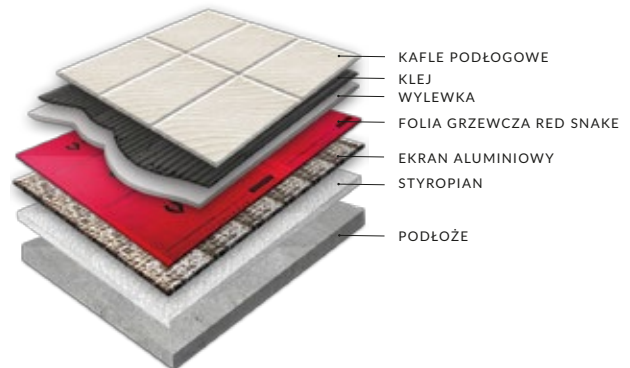
SCHEMAT UŁOŻENIA NA PODŁODZE Z PŁYTKAMI
